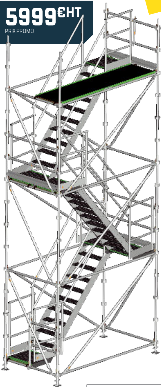
Modèle présenté : 6,00 m hauteur plancher Schéma non contractuel.
