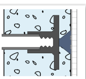
Entre banches avec aimant
