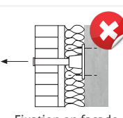
Fixation en façade
