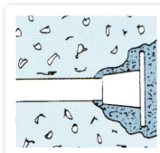
Réhabilitation platine encastrée
