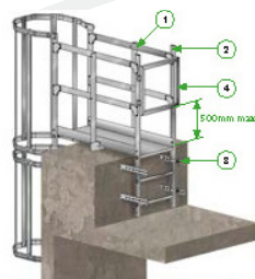
PALIER DE SORTIE POUR REDESCENTE D'ACROTÈRE
