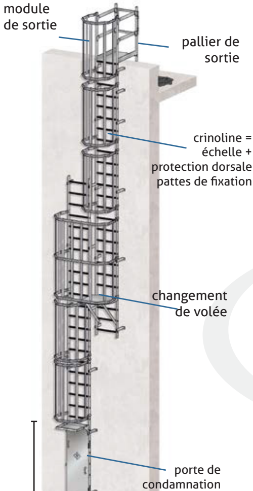
PALIER DE SORTIE POUR REDESCENTE D'ACROTÈRE
