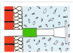
Mur composé Longueur réglable
